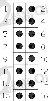
HUB75
