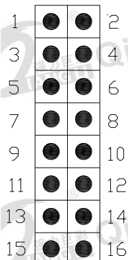
HUB75
